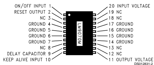
20-Pin SO Package
